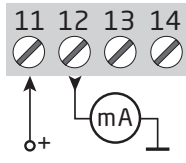
2-провод. передатчик (Пассивный выход)
