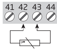
RTD, 2-проводн. сх.
